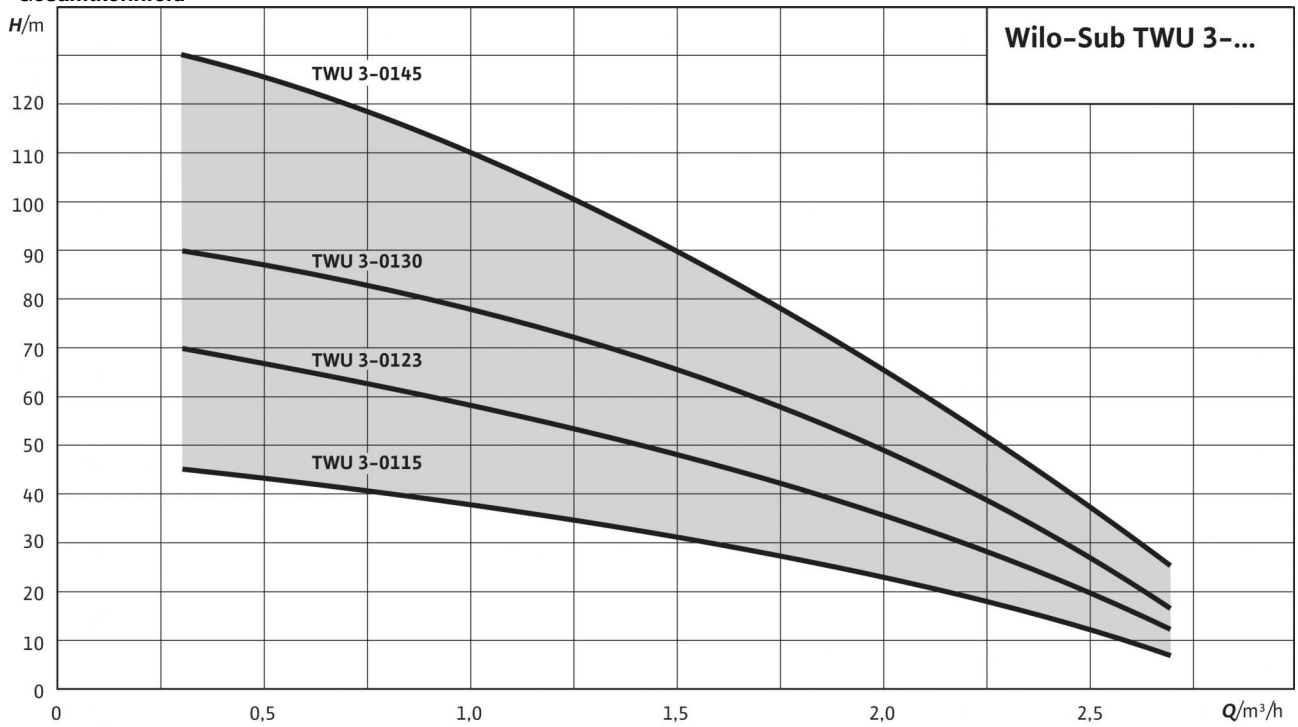
Gesamtkennfeld
